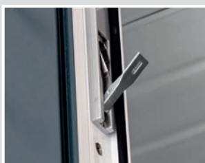
Kantregel för att låsa det fasta portbladet (uppe och nere)
